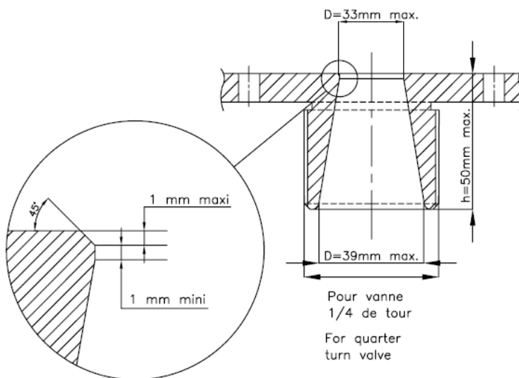
Dessin 255-10 Tekening 255-10
